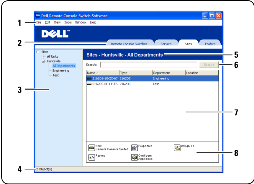
图 3.1: Explorer 窗口
